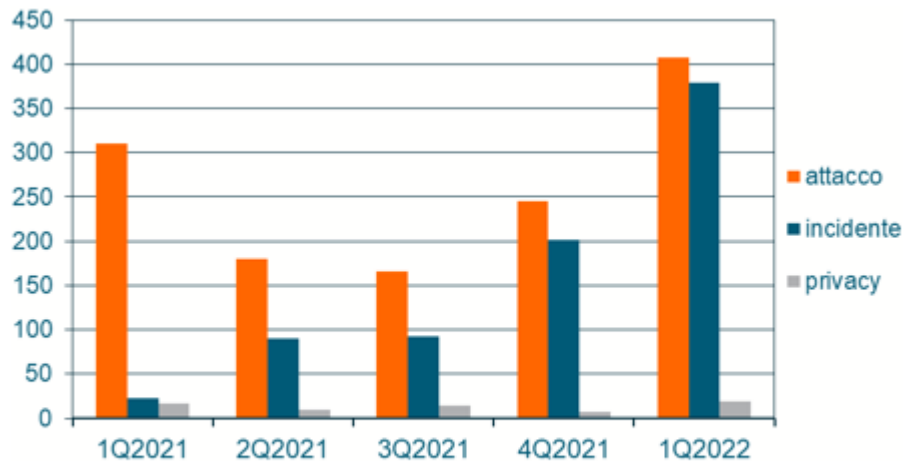
Figura 6 - Numero di attacchi, incidenti e violazioni privacy nel 2021, 1Q2022 in Italia
